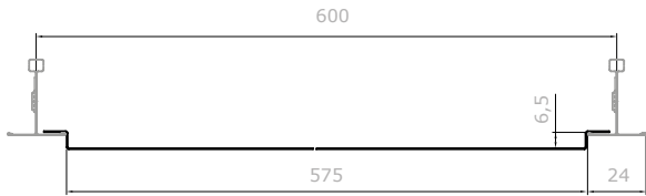
TEGULAR-24 A6 90°
