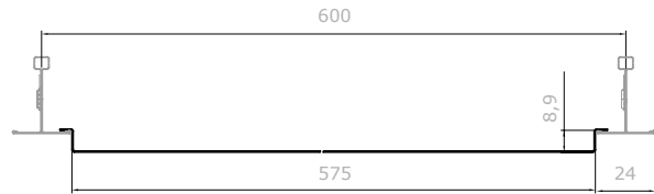
TEGULAR-24 A8 90°
